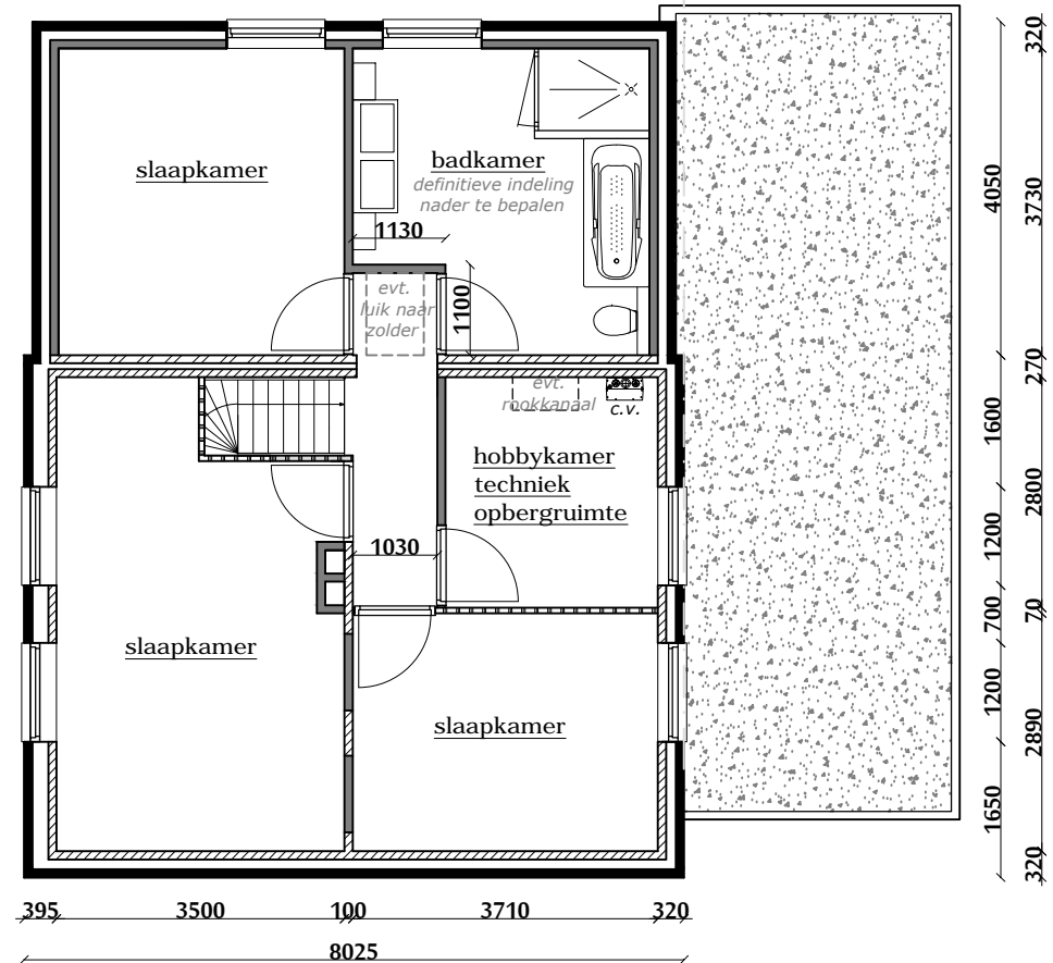
VERDIEPING NIEUW
